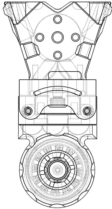
TOP
